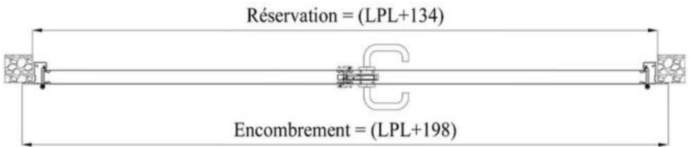
Coupe horizontale
