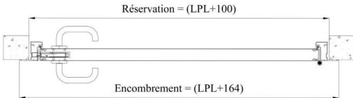
Coupe horizontale
