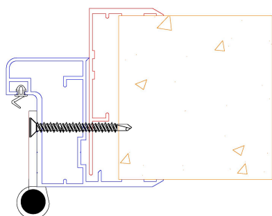
Fixation côté paumelle
