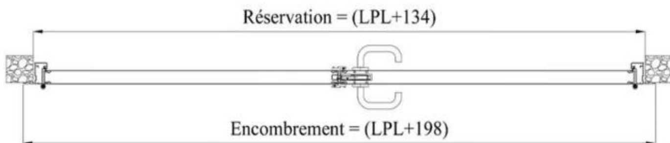
Coupe horizontale
