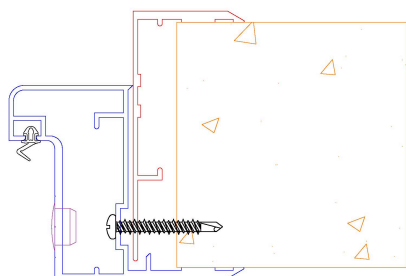
Fixation coté gâche.
