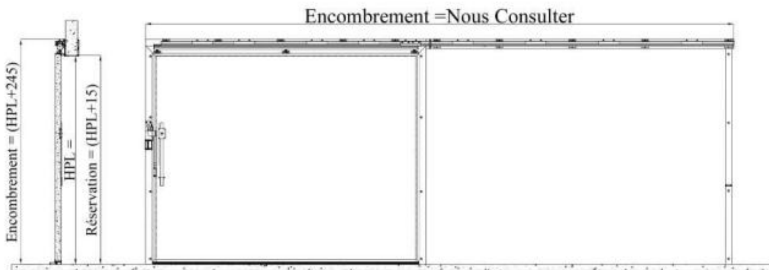
Coupe verticale
