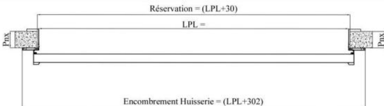
Coupe horizontale
