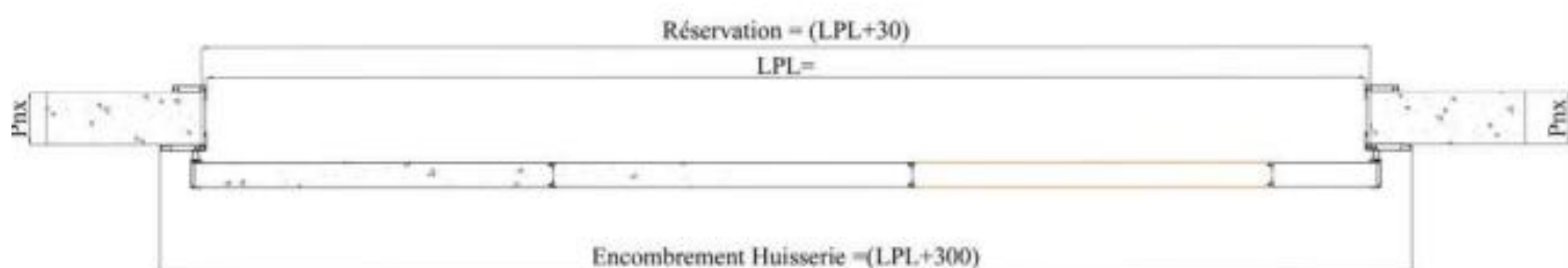
Coupe horizontale
