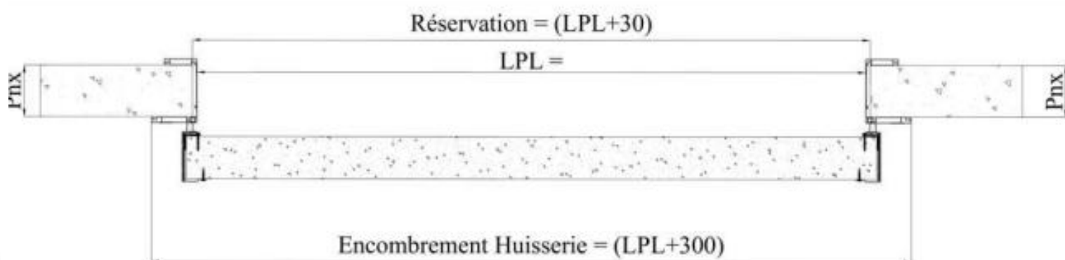
Coupe horizontale
