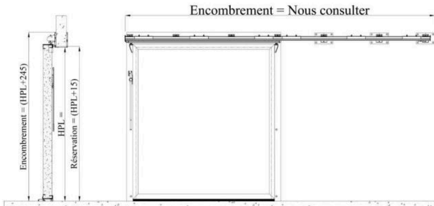
Coupe verticale
