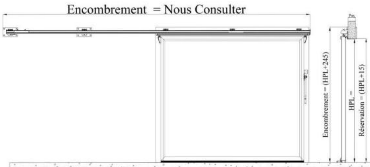
Coupe verticale
