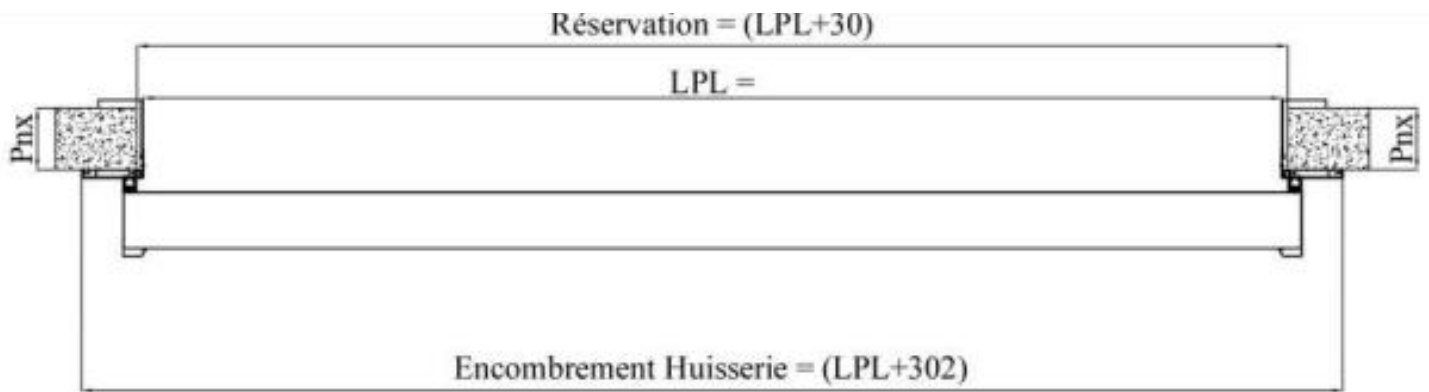
Coupe horizontale
