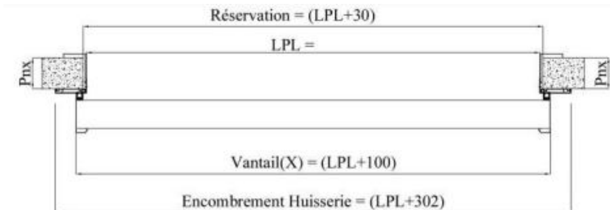
Coupe horizontale
