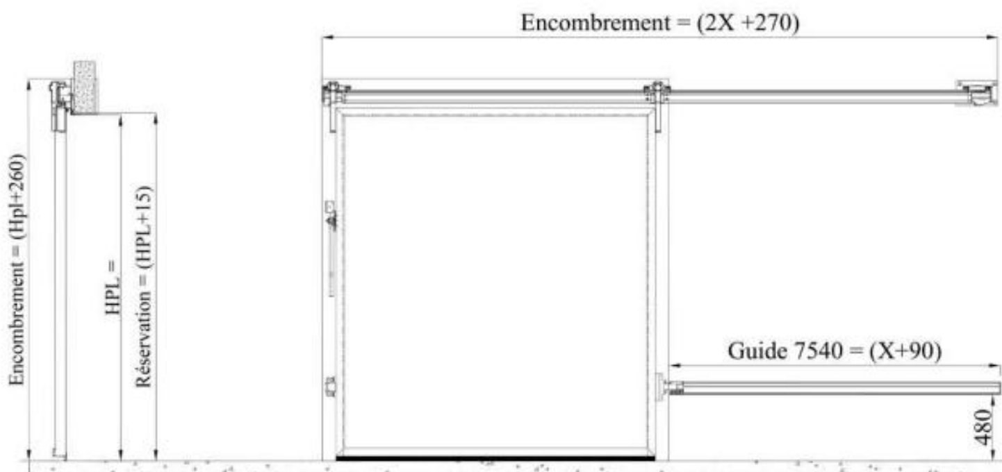
Coupe verticale
