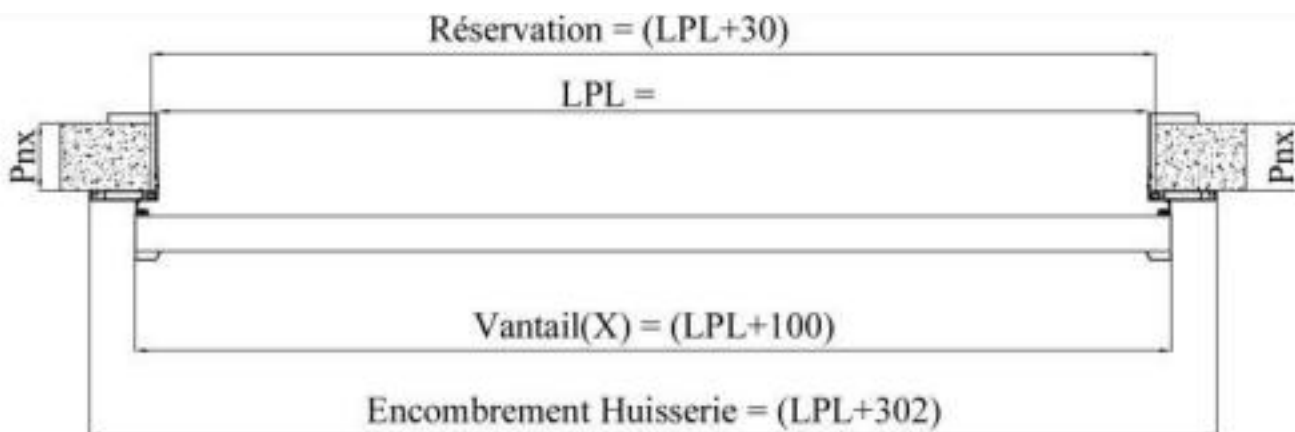
Coupe horizontale
