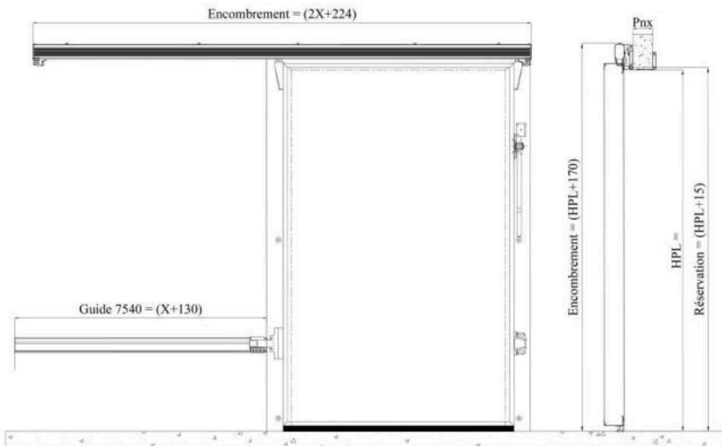
Coupe verticale
