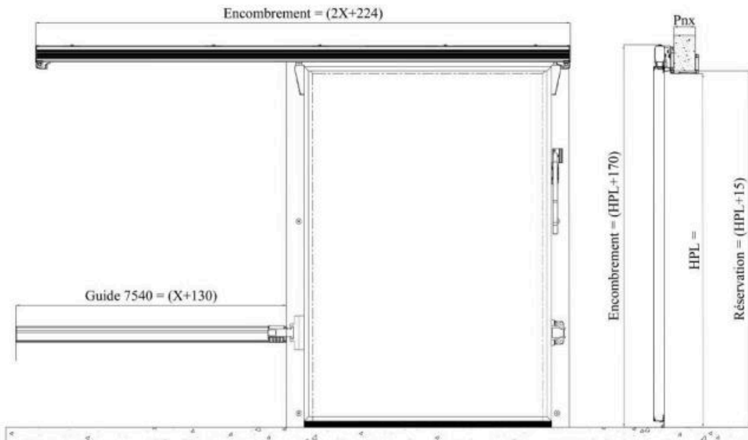
Coupe verticale
