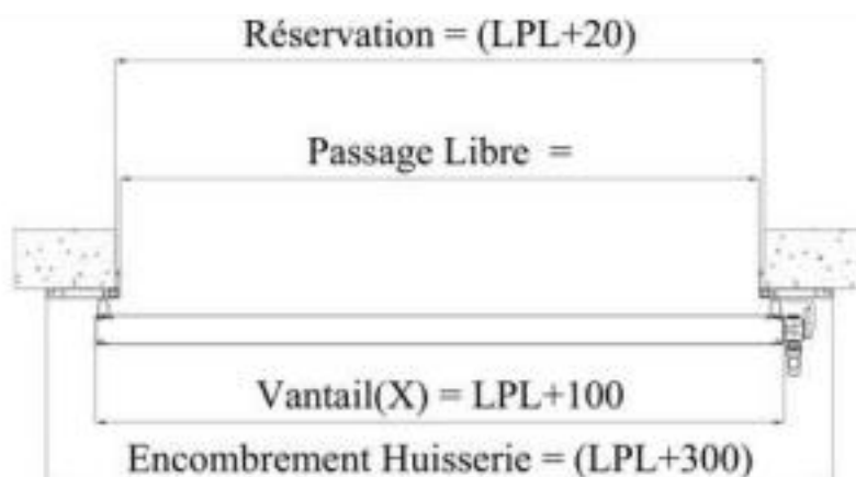
Coupe horizontale
