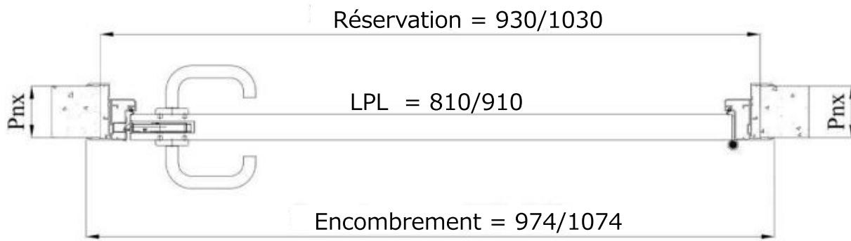
coupe horizontale
