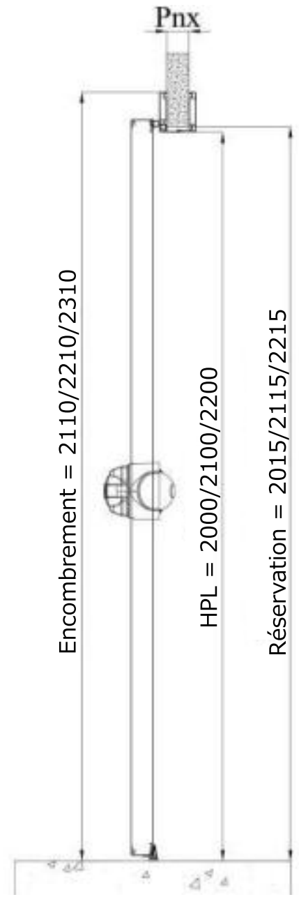
coupe verticale
