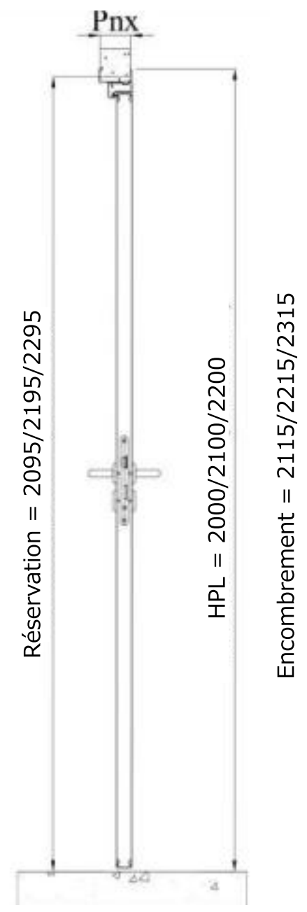
coupe verticale
