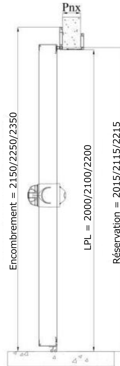
coupe verticale
