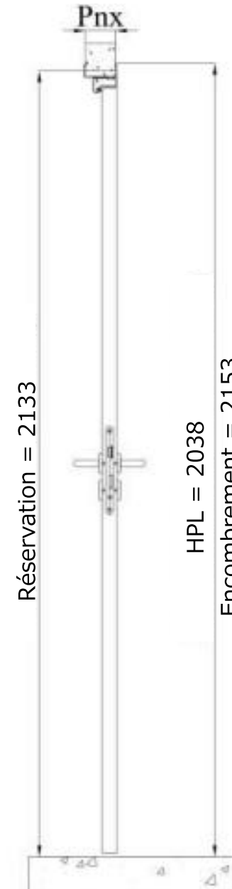
coupe verticale
