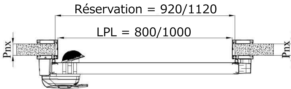
Trappe de visite froid positif 2
