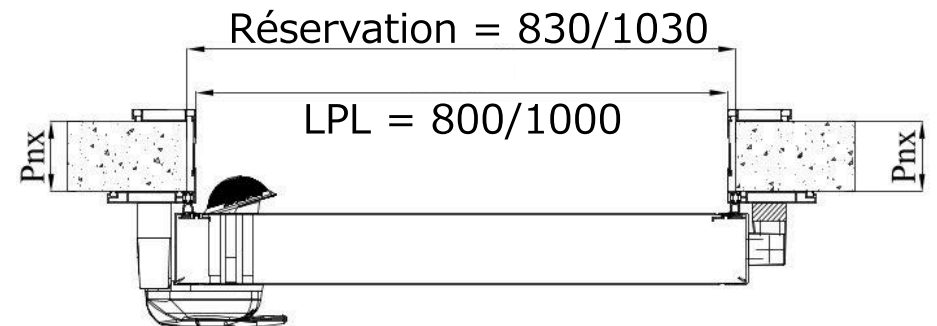
Trappe de visite froid négatif 3
